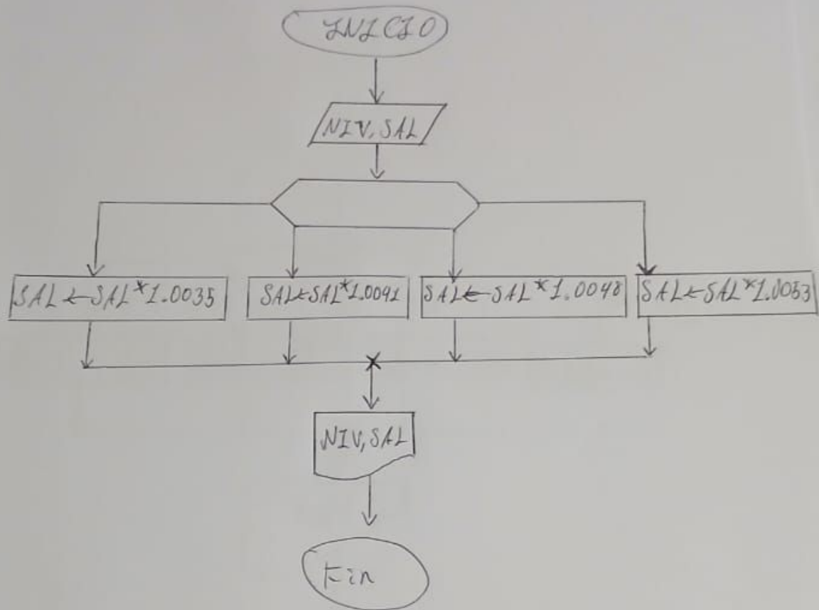
Diagrama de Flujos Programa 2.6
